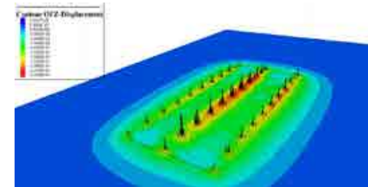
Figura 14. Asentamientos en condiciones actuales.
