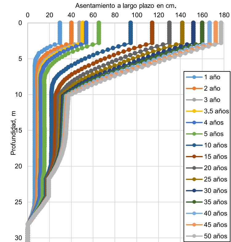
Figura 8. Asentamientos con el tiempo en función de la profundidad para el punto de monitoreo de mayor deformación.
