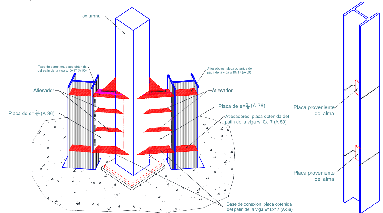
Figura 18. Conexión entre pilotes y columnas de la estructura y la unión entre secciones del pilote.
