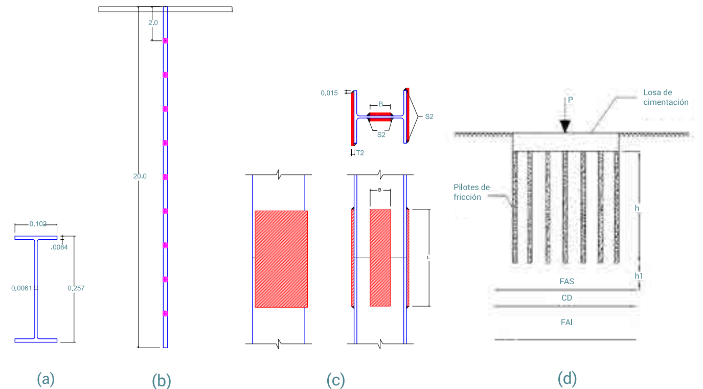
Figura 12. (a) Dimensiones del perfil, (b) Longitud del pilote, (c) Detalles de conexión en los tramos de los pilotes y (d) Esquema de pilotes de fricción.
